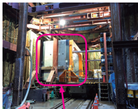
頂版推進中（中央がボックスカルバート）
