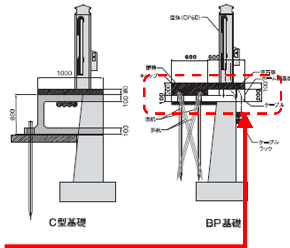
ホーム柵 基礎断面図 (新旧比較)
